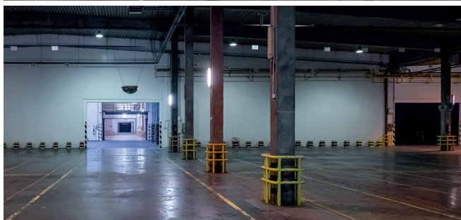
Hala magazynowa/produkcyjna o konstrukcji żelbetowej (słupy i dźwigary). Ściany zewnętrzne tradycyjne, warstwowe. Ocieplone i otynkowane tynkiem strukturalnym barwionym. W elewacji południowej (administracyjno-biurowa) fasada szklana o konstrukcji aluminiowej. Dach z blachy trapezowej ocieplony z powłokami bitumicznymi termozgrzewalnymi na dźwigarach żelbetowych. Schody żelbetowe monolityczne. Ściany wewnętrzne z cegły kratówki oraz w konstrukcji lekkiej. Posadzki w części produkcyjnej obiektu mają właściwości kwasoodporne, natomiast pozostałe są betonowe, zacierane, utwardzone.
